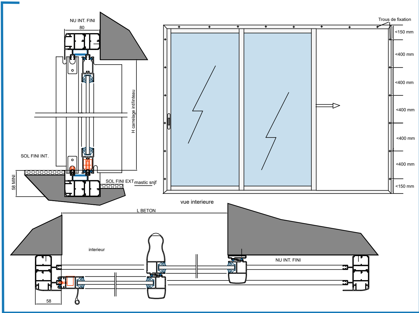
Montant renforcé
