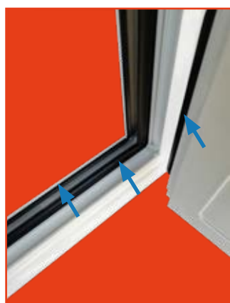
3 barrières d'étanchéité
