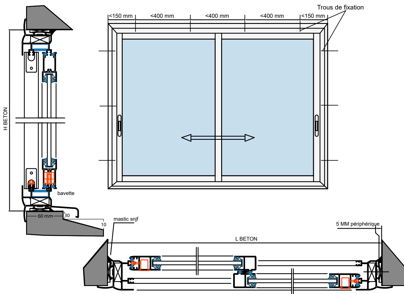
Brosse d'étanchéité
