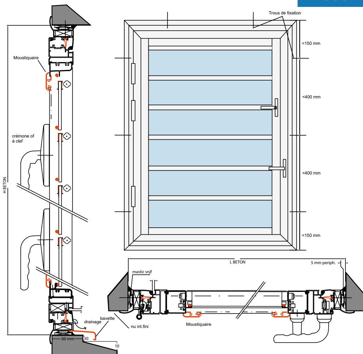
3 barrières d'étanchéité
